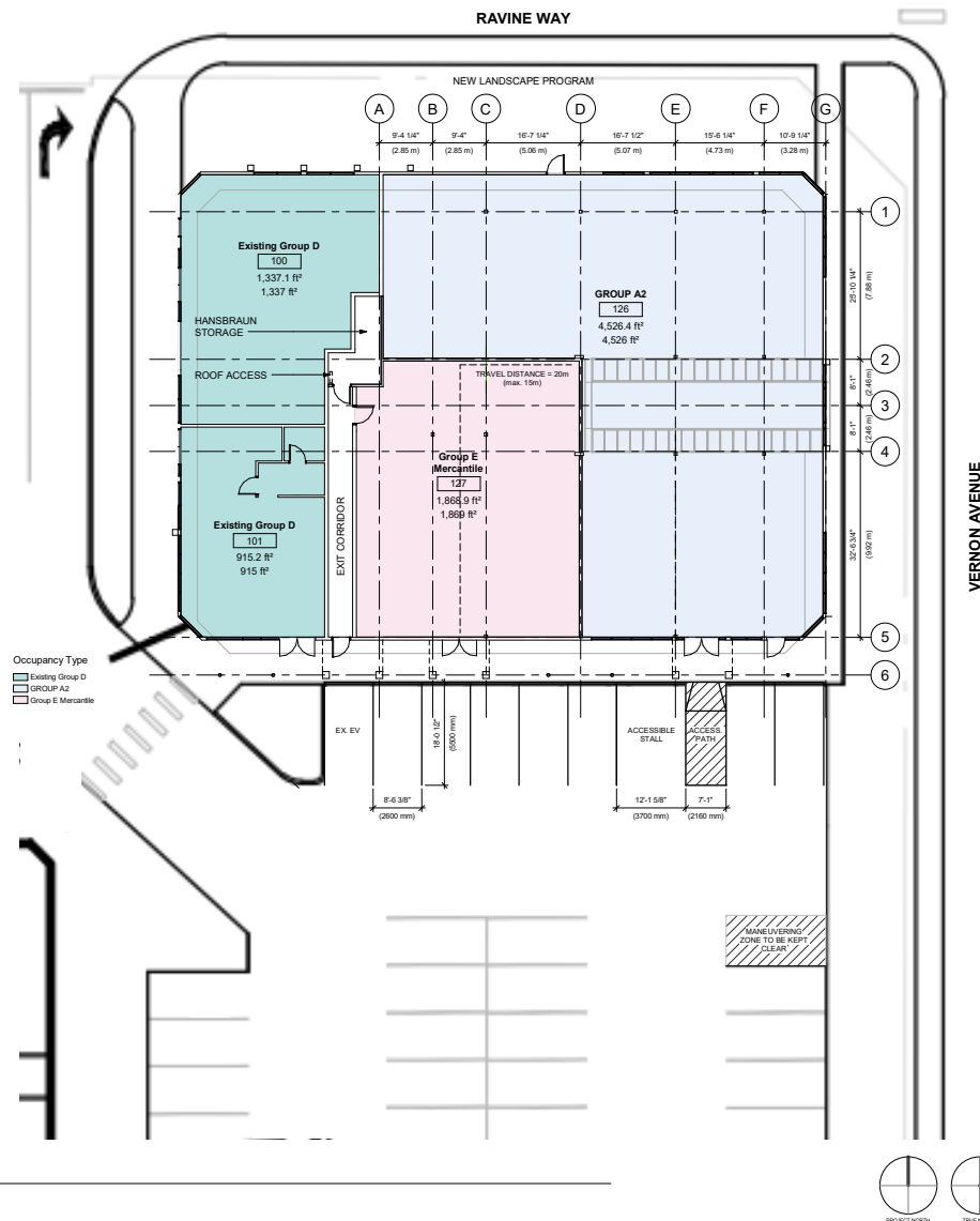
2 FLOOR PLAN A110 SCALE: 1" = 10'-0"
